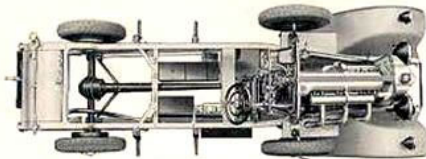
Fahrgestell (Draufsicht)
