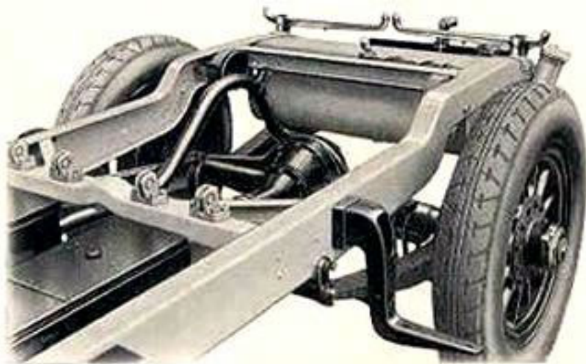
Rahmenende, Hinterachse
